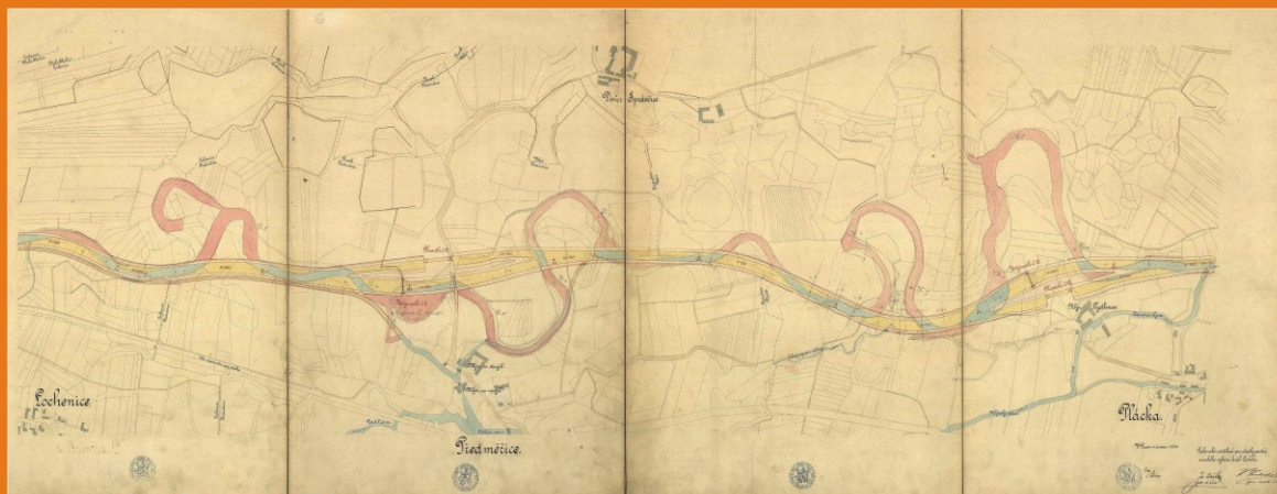
Situace plavebního stupně Předměřice a Plácka, 1904
