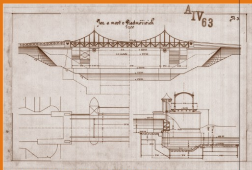
Typový návrh jezu a mostu v Předměřicích nad Labem, 1904
