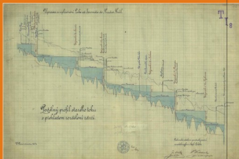
Podélný profil Labe v úseku Hradec Králové - Jaroměř s přehledem nových jezů, 1904
