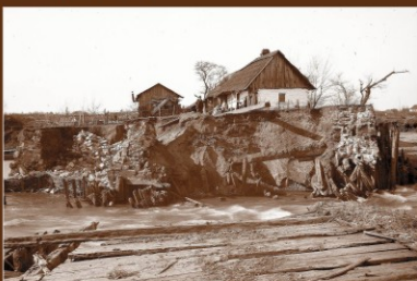
Pohled na zřícený pevný jez z levého břehu, 3. 3. 1918
