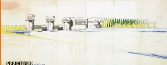
Návrh arch. Josefa Stěpánka - pohled na jez a vodní elektrárnu z horní vody, 1948
