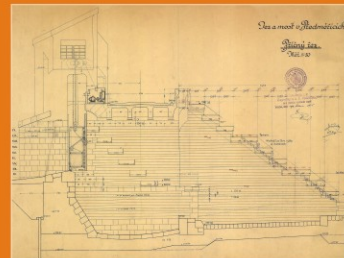
Příčný řez jezovým polem, 1915
