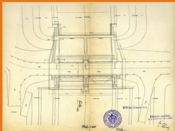
Situace nového jezu, 1914
