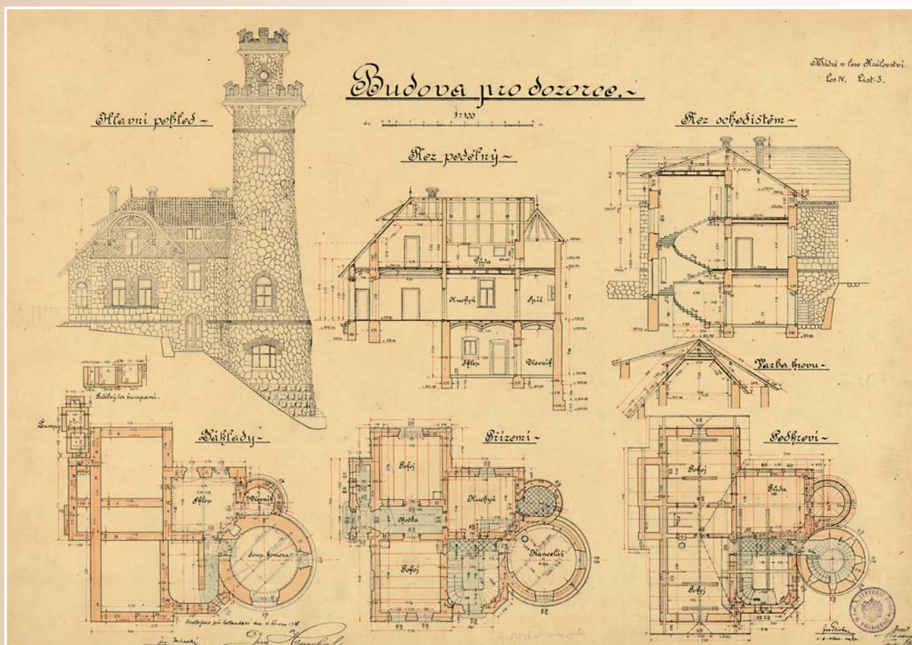
Původní projektová dokumentace - dům hrázného
