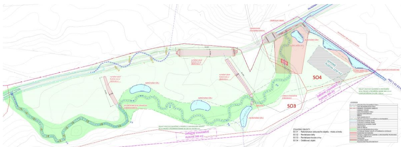
Situace revitalizovaného koryta, nových tůní, rozdělovacího objektu a upraveného hlavního odvodňovacího zařízení
