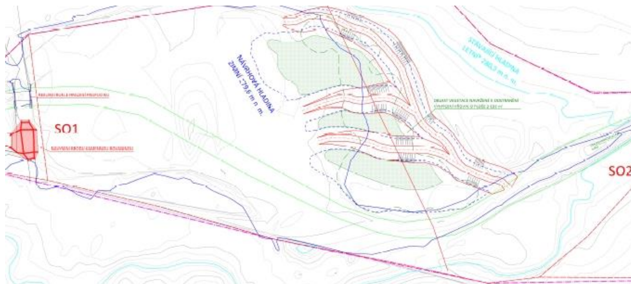
Situace zvýšeného brodu a delty
