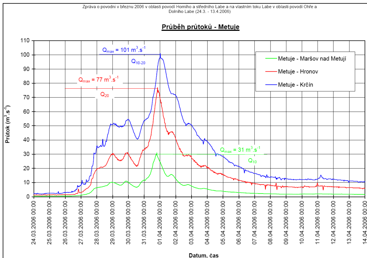
Obr. 2.1 Průběh průtoků povodní 2006 - Metuje
