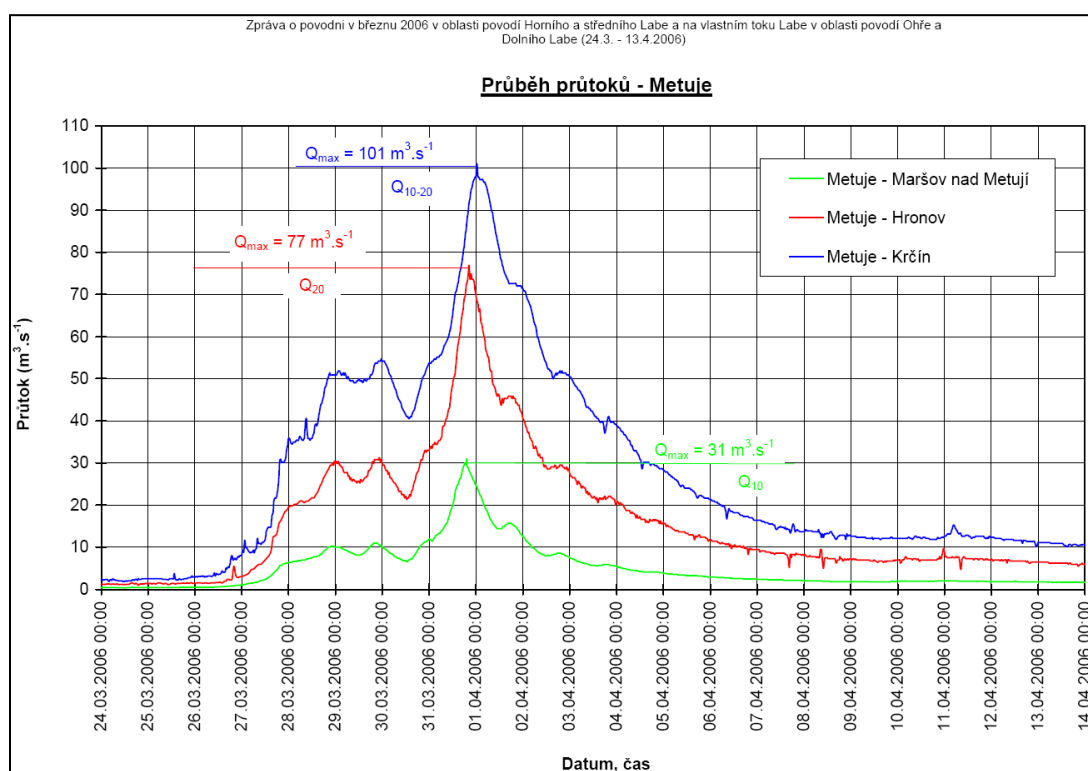
Obr. 2.1 Průběhy průtoků povodeň 2006 - Metuje
