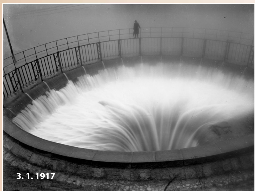
Pravý šachtový přeliv před kulminací
